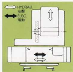
Extra wheel hub 額外砂輪法蘭
